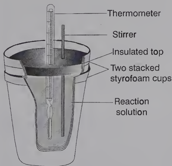
Figure 10.3 Simple Calorimeter (Rae Déjur)
