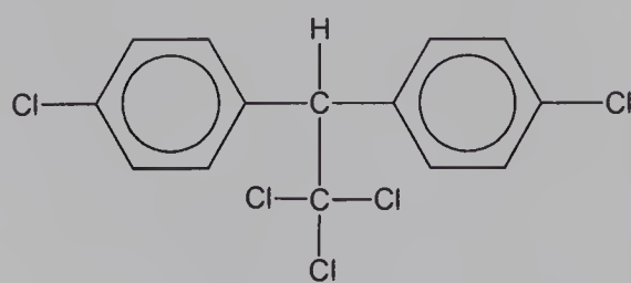
DDT
