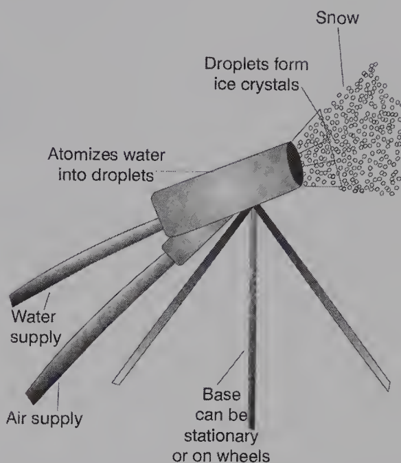
Figure 9.8 Snow Gun (Rae Déjur)
