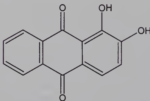
Alizarin
