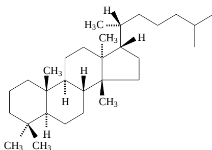
5\alpha -euphane 5\alpha , 13\alpha , 14\beta , 17\alpha -lanostane
