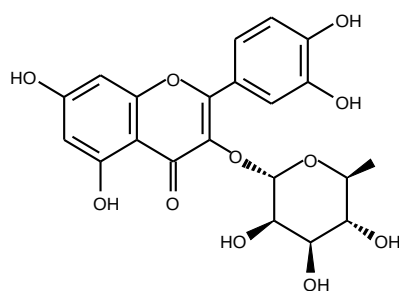
29-34 quercitrin
