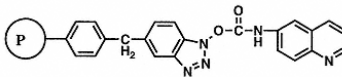
Fig. 2.20. Polymeric Benzotriazole-6-AQ.
