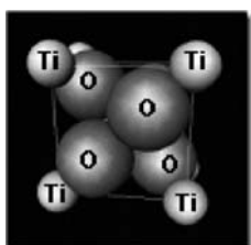
Rutile ( \text{TiO}_2 )
