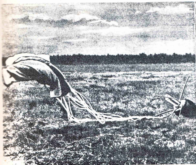
СПУСКАЕМЫЙ АППАРАТ «ЛУНЫ-16» ВО ВРЕМЯ ИСПЫТАНИЙ. На правом снимке видны надувные чехлы с антеннами
