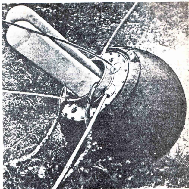
СПУСКАЕМЫЙ АППАРАТ «ЛУНЫ-16» ВО ВРЕМЯ ИСПЫТАНИЙ. На правом снимке видны надувные чехлы с антеннами
