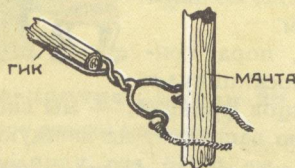
С ПОМОЩЬЮ ТАКОЙ ПРОВОЛОЧНОЙ ВИЛКИ ГИК СОЕДИНЯЕТСЯ С МАЧТОЙ
