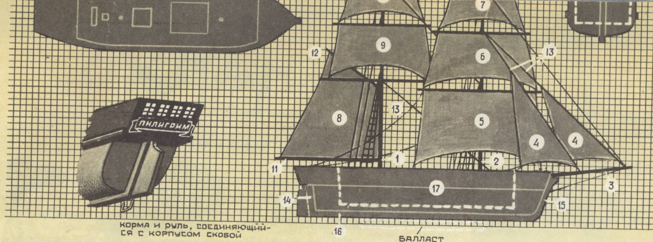
БАЛЛАСТ
