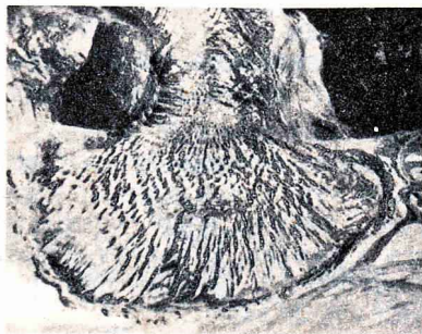
Кажется, застывшие потоки образованы особой горной породой. На самом деле — это лед, одно из состояний воды.
