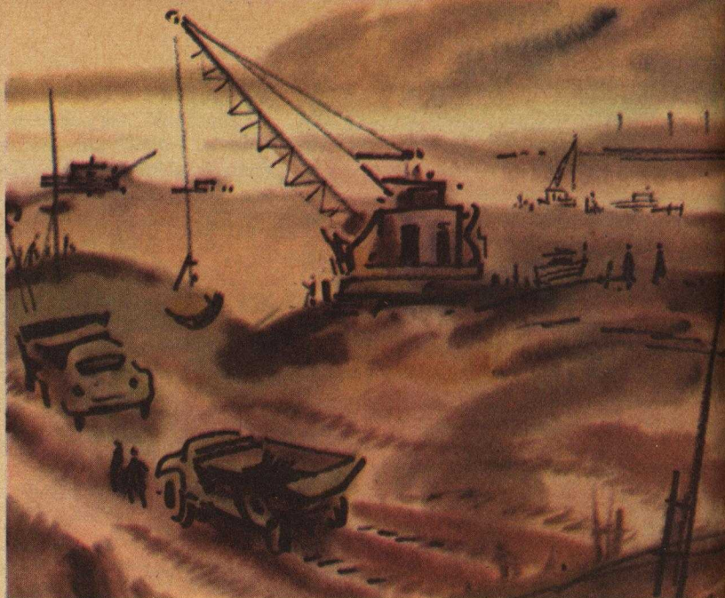
Строительство Копет-Дагского водохранилища
