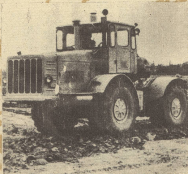
Трактор К-701
