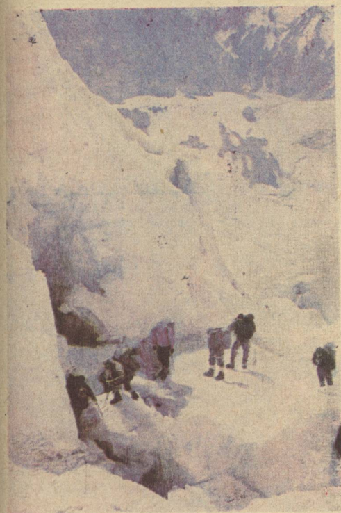
В лабиринте трещин ледника Бивачный
