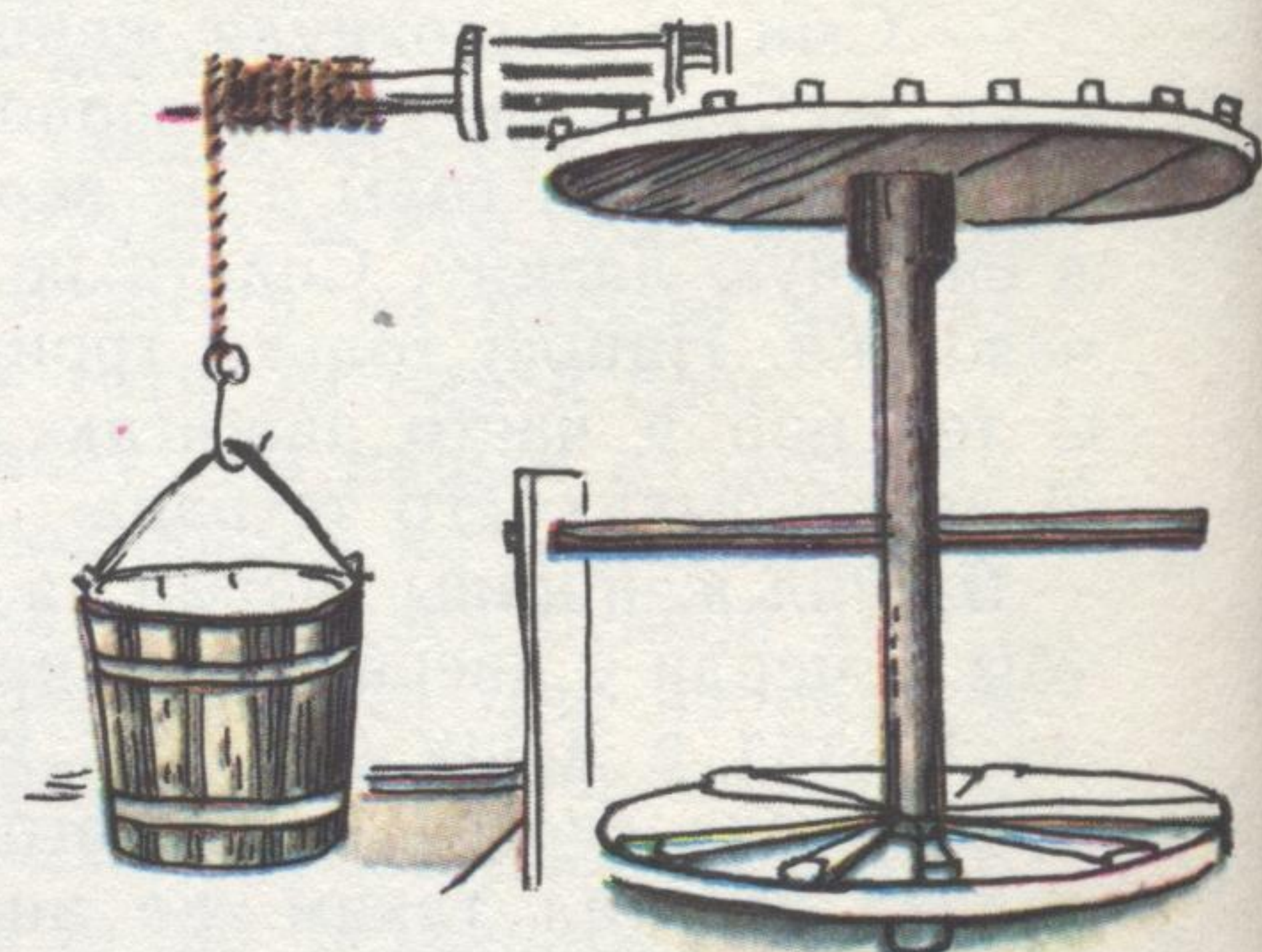
Ворот и винтовой деревянный домкрат
