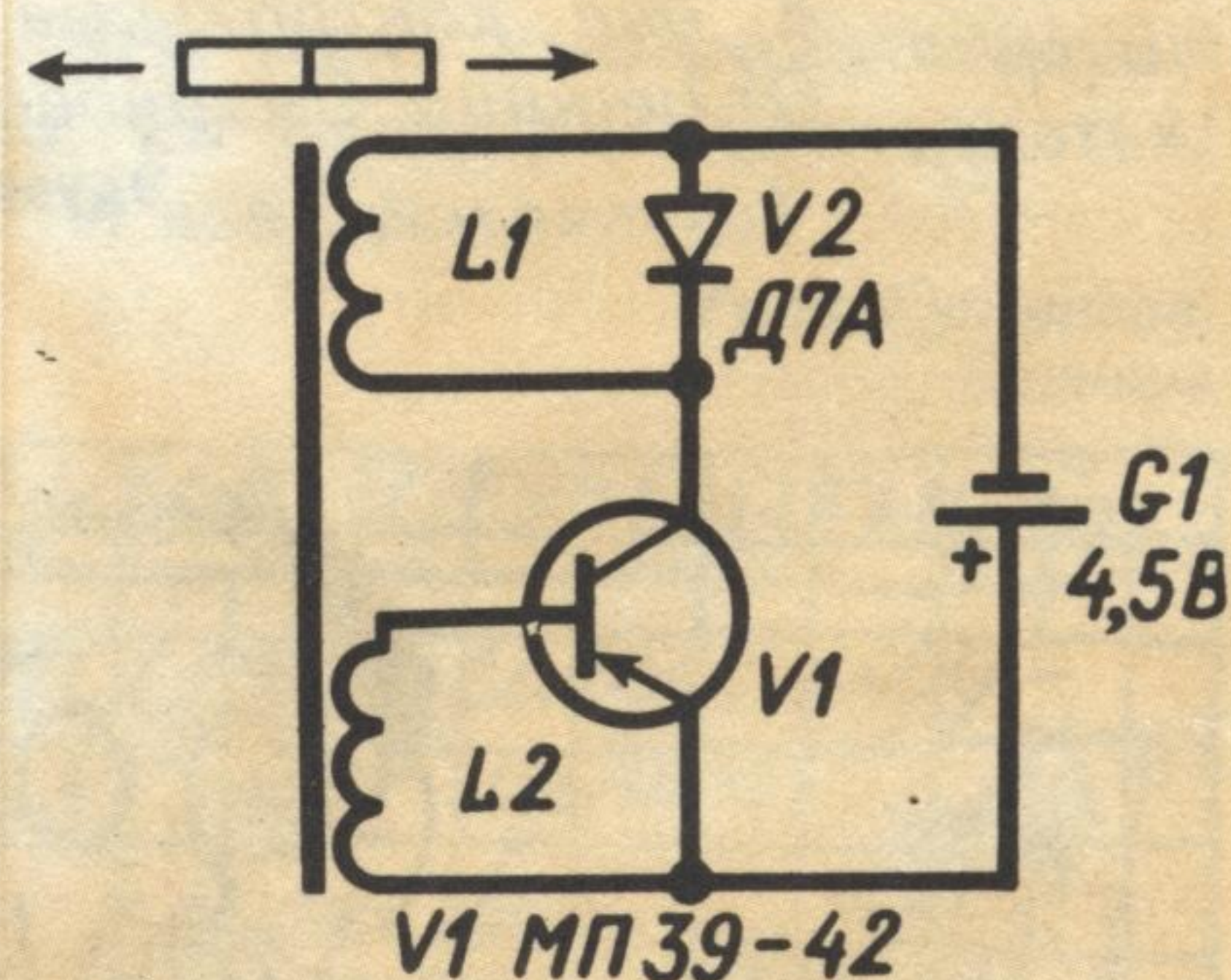
Рис. 4. Принципиальная схема электронной части качелей
