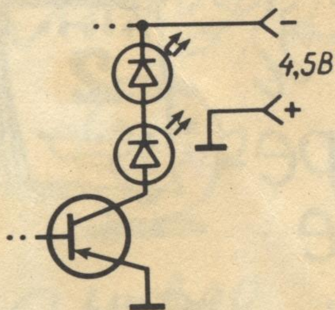
Рис. 2. Принципиальная схема включения светодиодов в устройство подсветки елки
