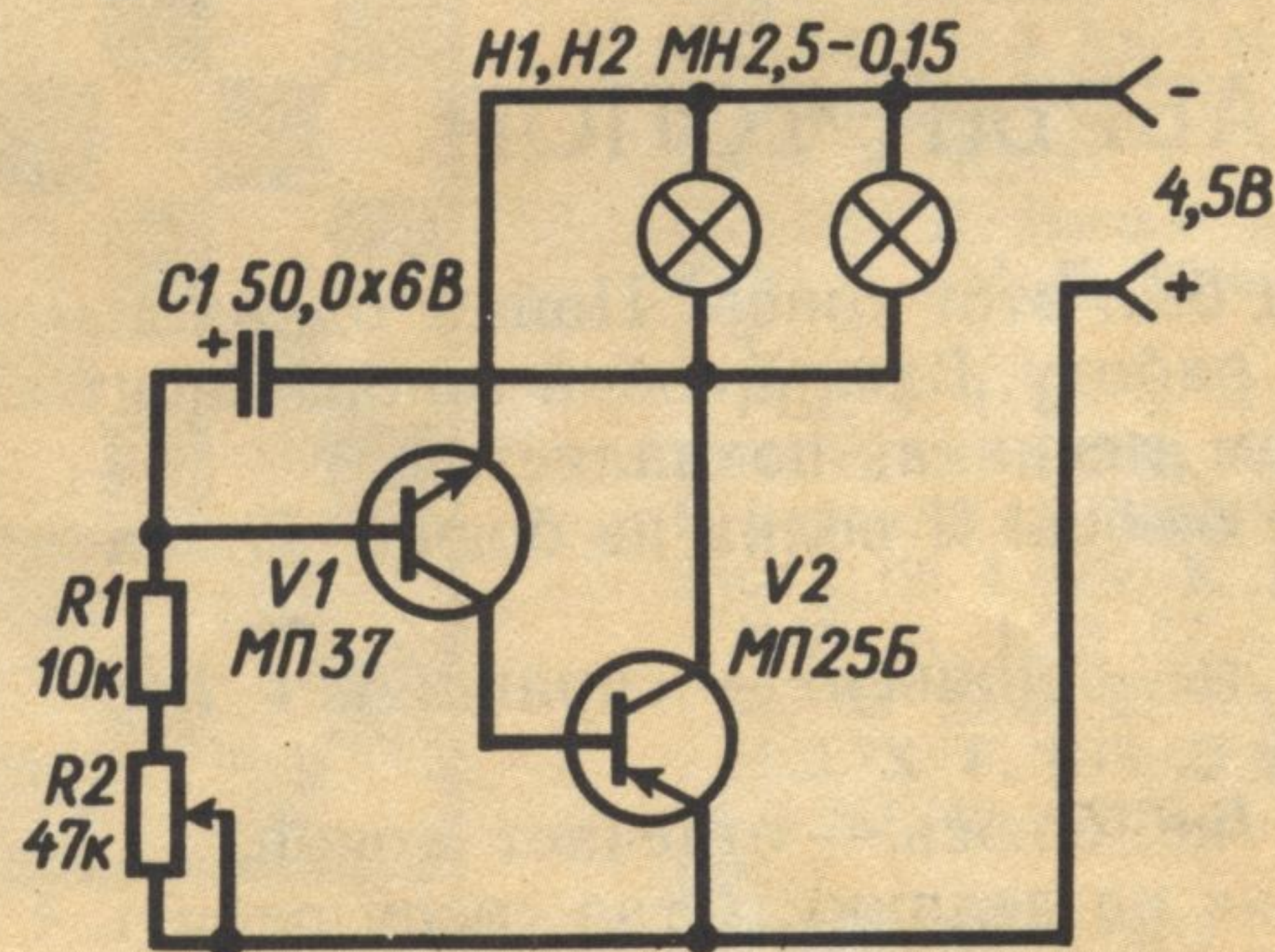
Рис. 1. Принципиальная схема устройства периодической подсветки новогодней елки
