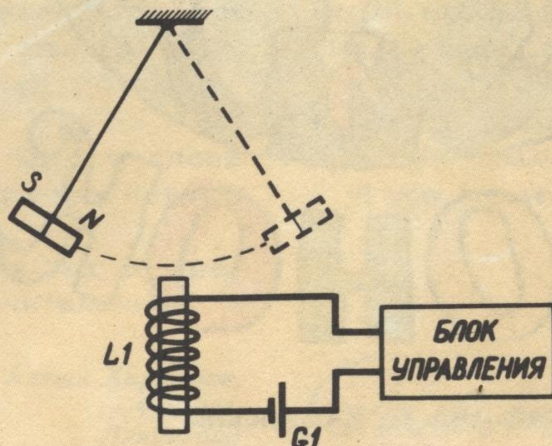
Рис. 3. Схема электронных качелей
