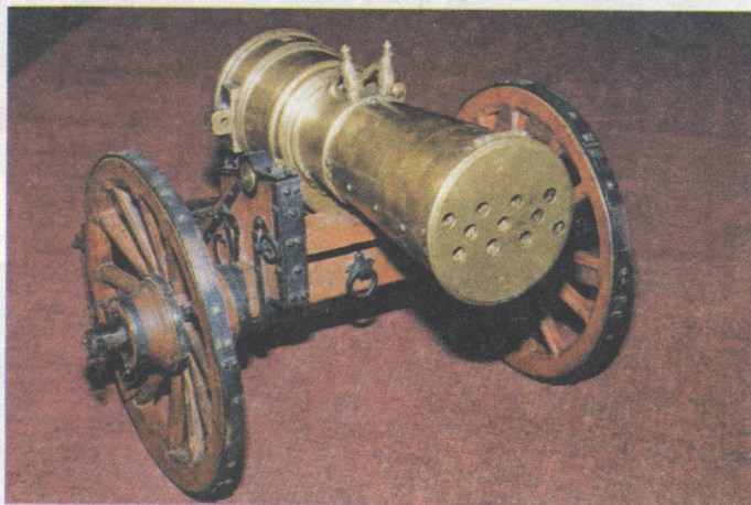
11-канальная казнозарядная опытная картечница. Конец XVIII века. (1/5 натуральной величины). Орудие является системой залпового огня с механизмом горизонтальной наводки для поворота ствола вокруг продольной оси.
