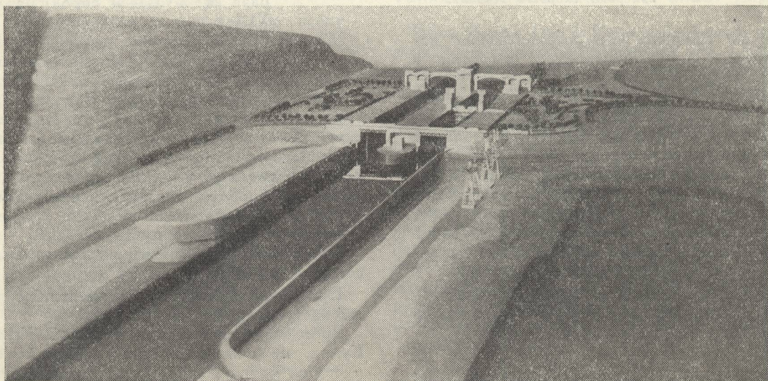
Здесь вы видите шлюз — часть макета Куйбышевского гидроузла. Макет сделан из алюминия, в 1/500 натуральной величины и находится сейчас в павильоне СССР на Ньюйоркской выставке.
