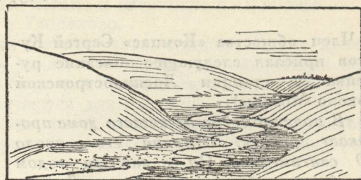
Рис. 4. Старая река.
