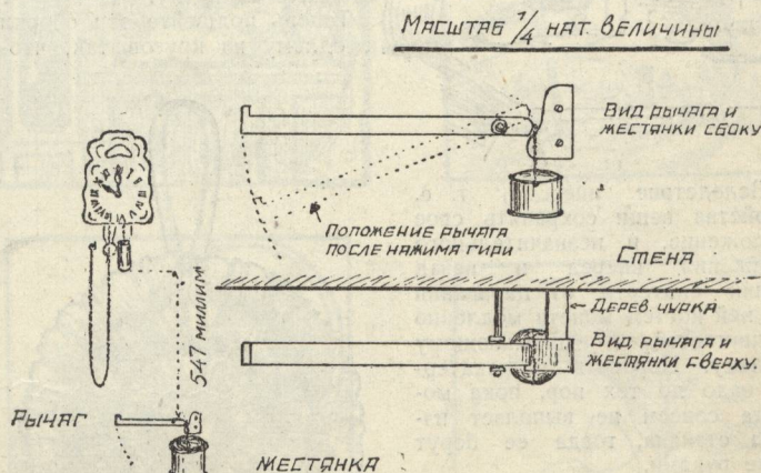
Схема вторая — без электрического звонка.
