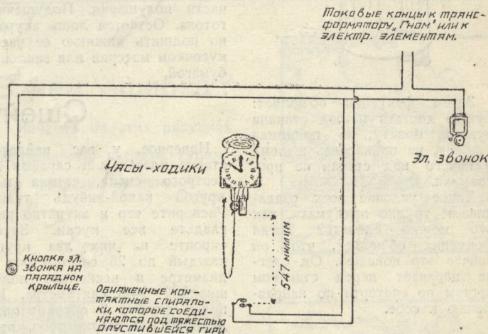
Схема, по которой можно построить электрический будильник собственной конструкции
