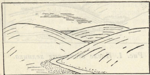
Рис. 3. Зрелая река.
