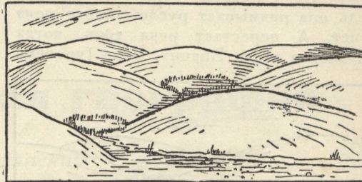
Рис. 1. После стаивания ледника.
