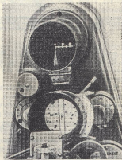
Микрофотометр — очень чувствительный прибор. Он помогает изучать самые далёкие звёзды. Здесь вы видите микрофотометр университетской обсерватории, а рядом — то, что он показывает. Тёмные кружочки в нижнем окошечке — изображения звёзд на фотопластинке. Астроном навёл звезду на щель в приборе. Тотчас в верхнем окошечке световая стрелка скользит по шкале к делению, соответствующему яркости звезды.
