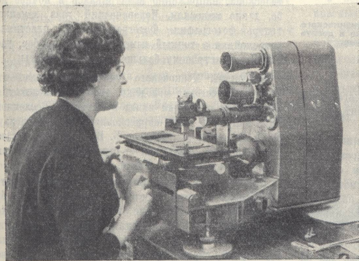
Микрофотометр — очень чувствительный прибор. Он помогает изучать самые далёкие звёзды. Здесь вы видите микрофотометр университетской обсерватории, а рядом — то, что он показывает. Тёмные кружочки в нижнем окошечке — изображения звёзд на фотопластинке. Астроном навёл звезду на щель в приборе. Тотчас в верхнем окошечке световая стрелка скользит по шкале к делению, соответствующему яркости звезды.
