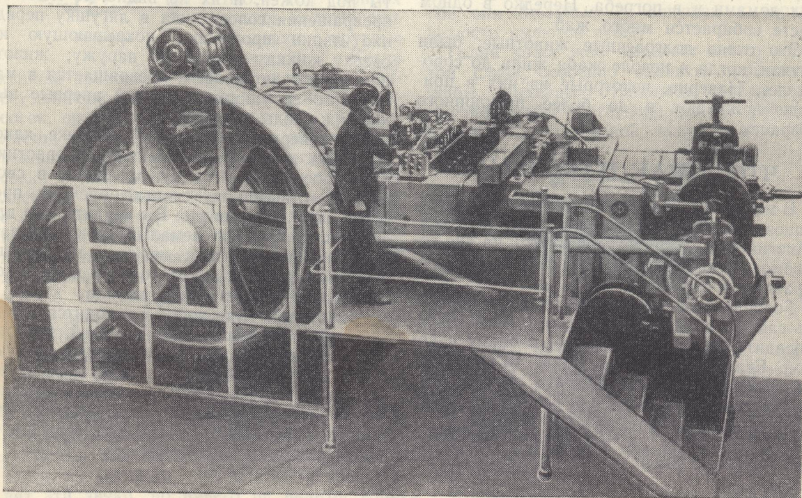
Эта штамповочная машина обрабатывает холодную сталь. Она делает шестьдесят гаек в минуту.
