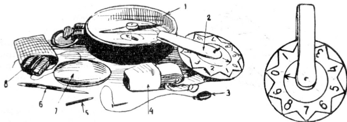
Рисунок 2. (1 — компас; 2 — курвиметр; 3 — нитка для эклиметра; 4 — вымпел; 5 — теневая палочка для солнечного высотомера; 6 — теневая палочка для солнечных часов; 7 — лупа; 8 — секундомер).
