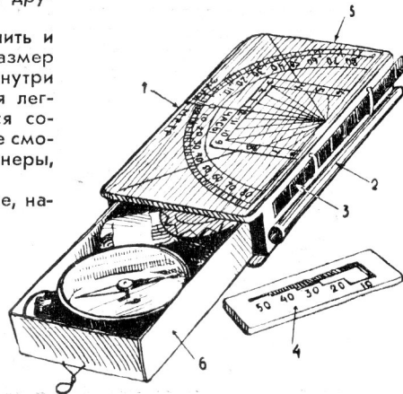
Рисунок 1. (1 — на этой стороне пенала расположен солнечный высотомер; 2 — трубочка; 3 — линейка дальнотмера; 4 — крышка с «лесенкой»; 5 — крышка с отверстием; 6 — коробочка с компасом, курвиметром и др.).
