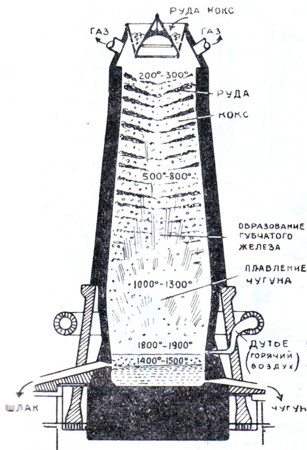
Разрез доменной печи.
