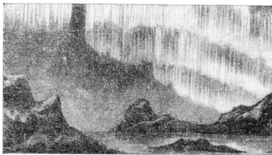
Под ударами летящих от Солнца частиц разреженные газы земной атмосферы начинают светиться, и в небе загорается полярное сияние.
