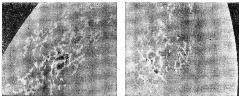
Близ края солнечного диска разыгралась буря, возникла группа пятен и факелов (правый снимок). Прошло несколько дней, пятна и факелы стали крупнее, буря, разыгрываясь, захватила обширную область (левый снимок). Благодаря вращению Солнца вокруг своей оси буря переместилась к противоположному краю солнечного диска.
