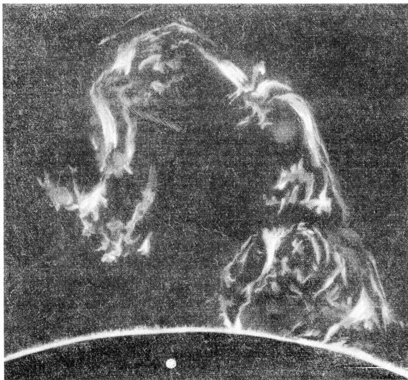
Гигантский выброс раскалённых газов на Солнце — протуберанец. Белая горошинка, нарисованная внизу для сравнения, — Земля.
