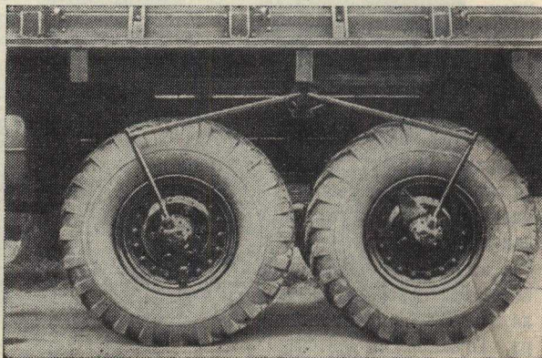
А это новость — устройство для подкачки шин. С таким устройством можно подкачать воздух в баллоны даже на ходу.
