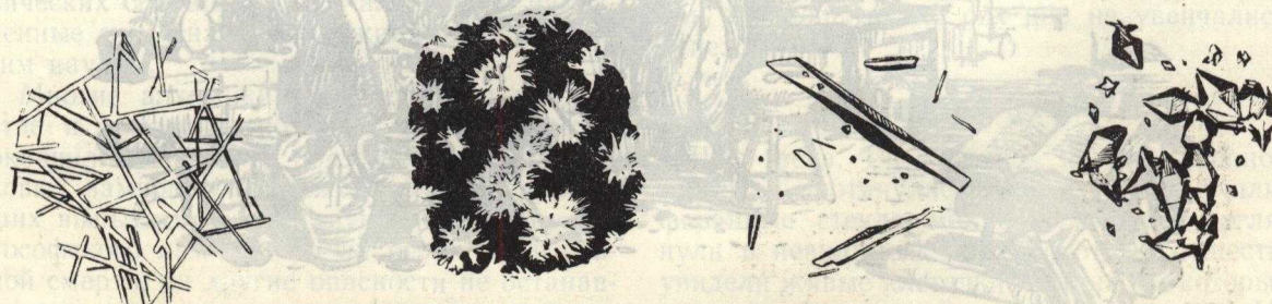
Вот как выглядят кристаллы различных ферментов. Ровненькие палочки слева — это кристаллы гексокиназы. Похожие на снежинки звездочки — кристаллы рибонуклеазы. Дальше идут кристаллы карбоксипептидазы и пепсина.
