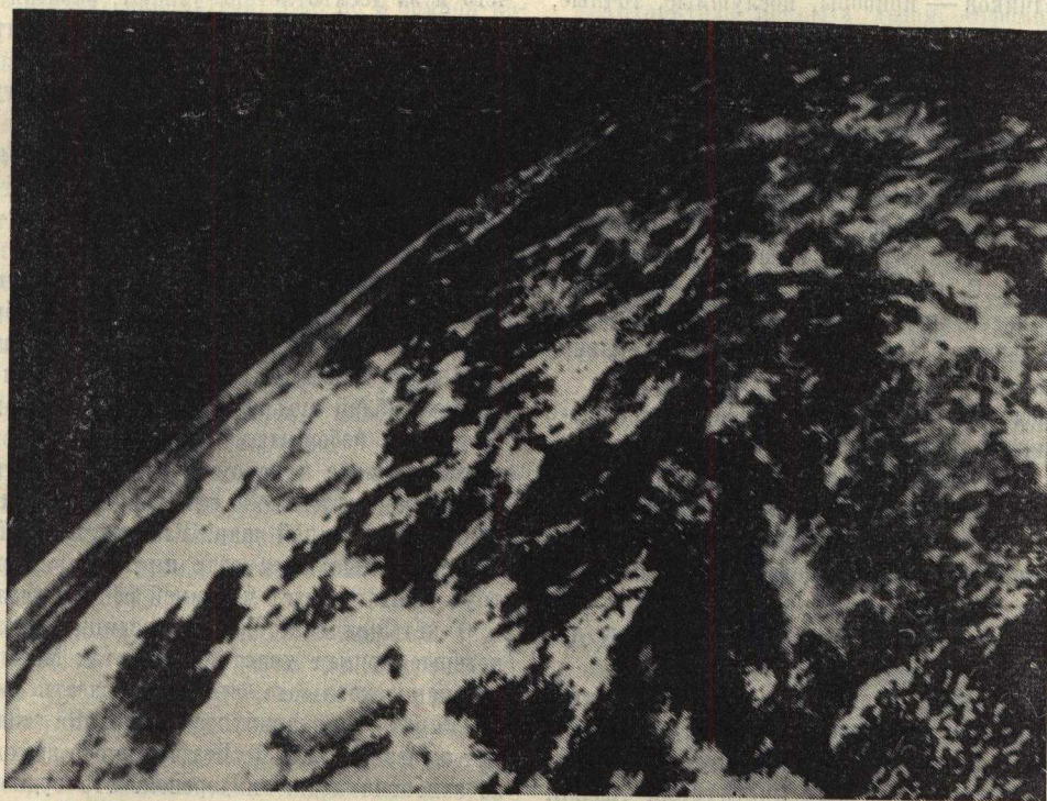
Эта фотография сделана ракетой с высоты 225 километров; она охватывает около полутора миллионов квадратных километров, и на ней отчетливо видна кривизна земной поверхности.
