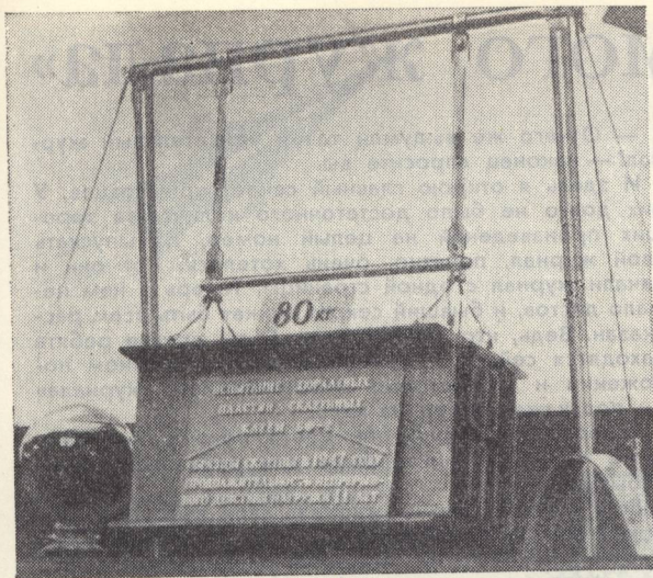
Вы видите здесь две дюралевые пластины (вертикальные), которые были в 1947 году склеены клеем БФ-2. Вот уже одиннадцать лет на них висит груз в 80 килограммов.
