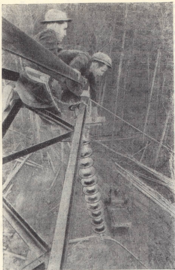
Последние гирлянды изоляторов, последние прогоны проводов остаются повесить на тридцатиметровые опоры, и ток пойдет по новой высоковольтной линии.
