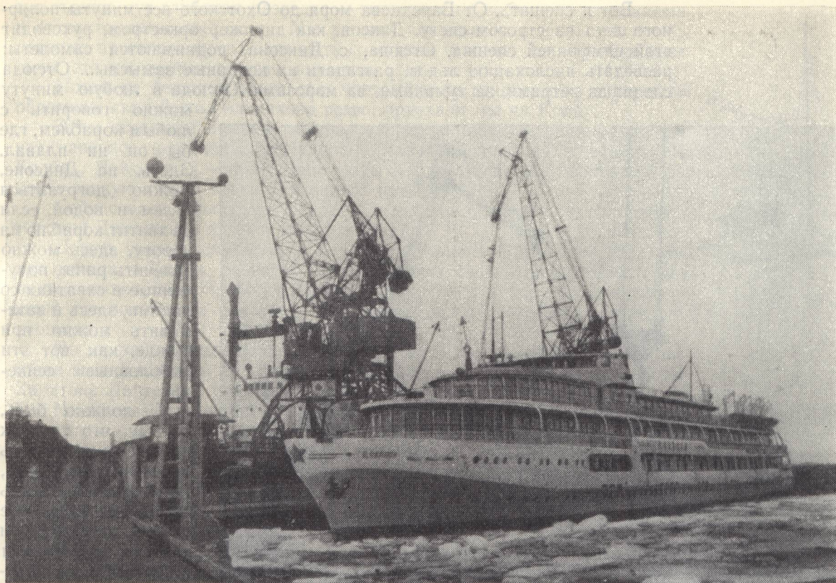
Причальный пирс порта Диксон оборудован мощными порталными кранами. Здесь одновременно могут разгружаться несколько морских кораблей.
