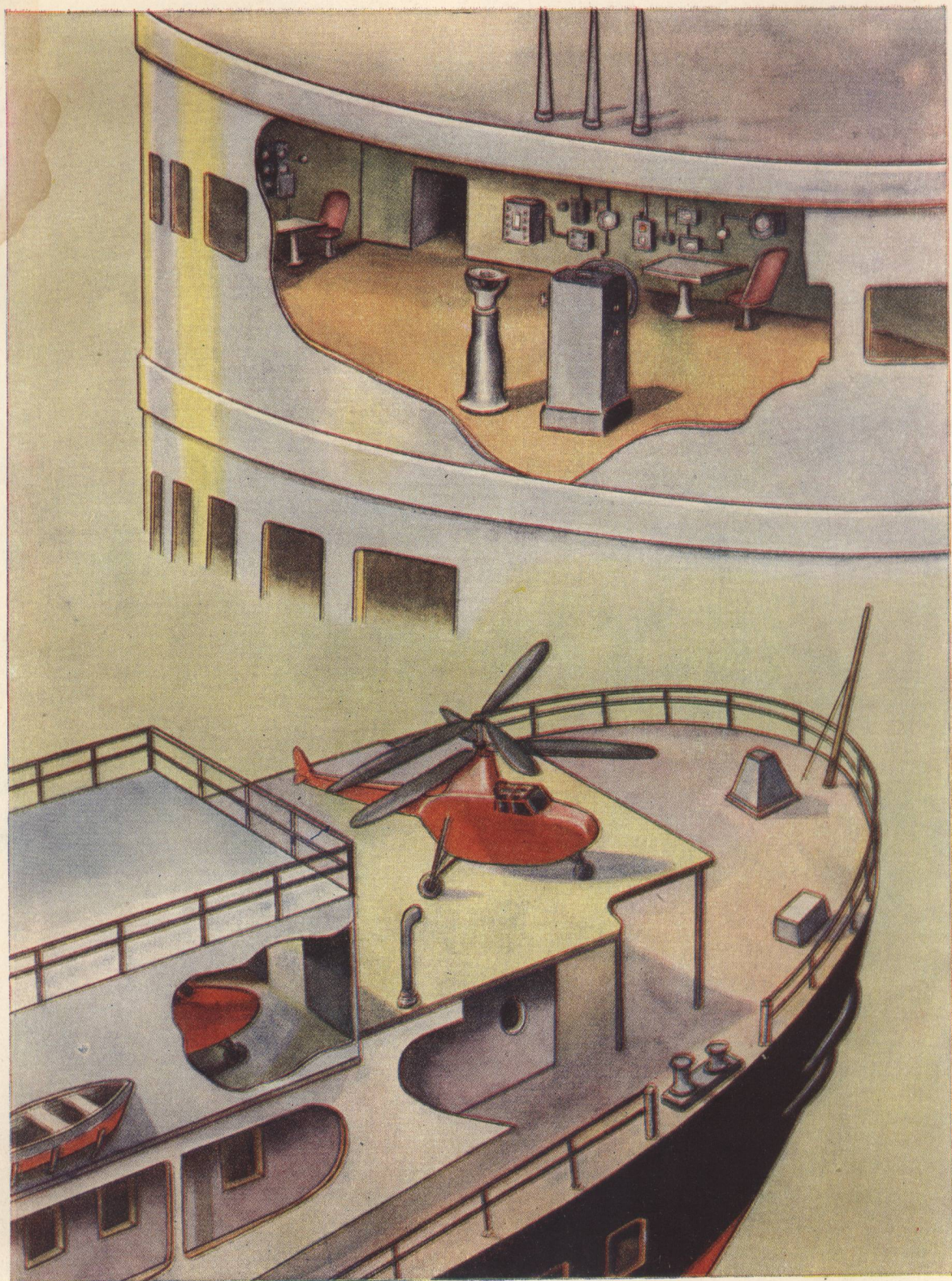
На верхнем рисунке — ходовая рубка атомного ледокола; внизу — кормовая часть корабля. На ней свободно размещаются два вертолета и ангар.
