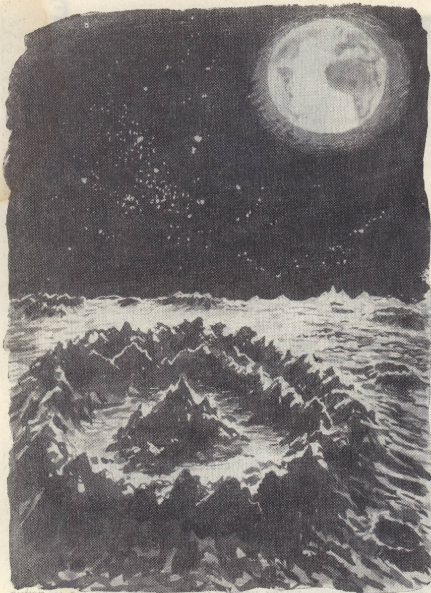
Ночи на Луне светлее земных. Диск «полной» Земли в тринадцать раз больше, чем лунный, а отраженного солнечного света Земля посылает Луне в восемьдесят раз больше, чем полная Луна Земле.
