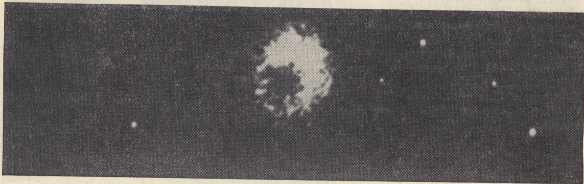
Так выглядела искусственная комета — вспышка натриевого облака, выпущенного второй межпланетной ракетой.
