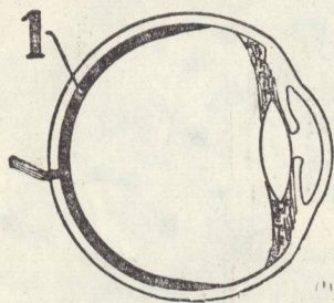
Сетчатка расположена на дне глаза. На этой схеме она помечена черным цветом.
