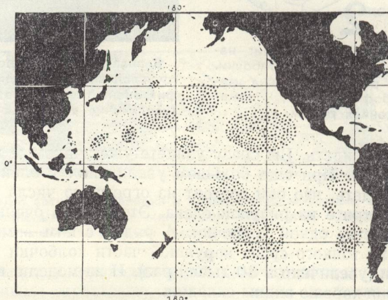
Это карта распространения «подводных клад». Густые точки показывают, где конкреции лежат вплотную, как на верхнем снимке.
