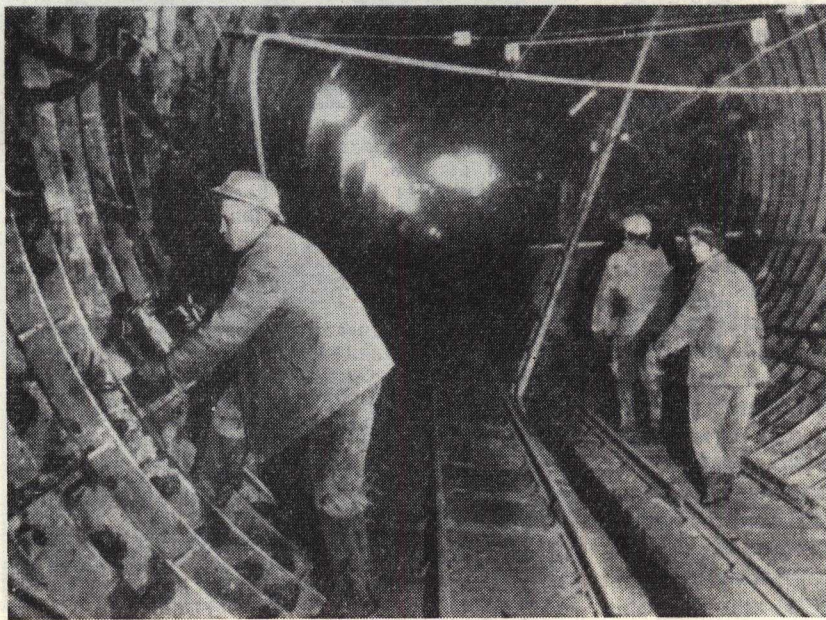
Вслед за щитом укладываются железобетонные кольца для крепления стенок тоннеля.
