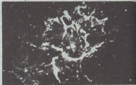
Крабовидная туманность.
