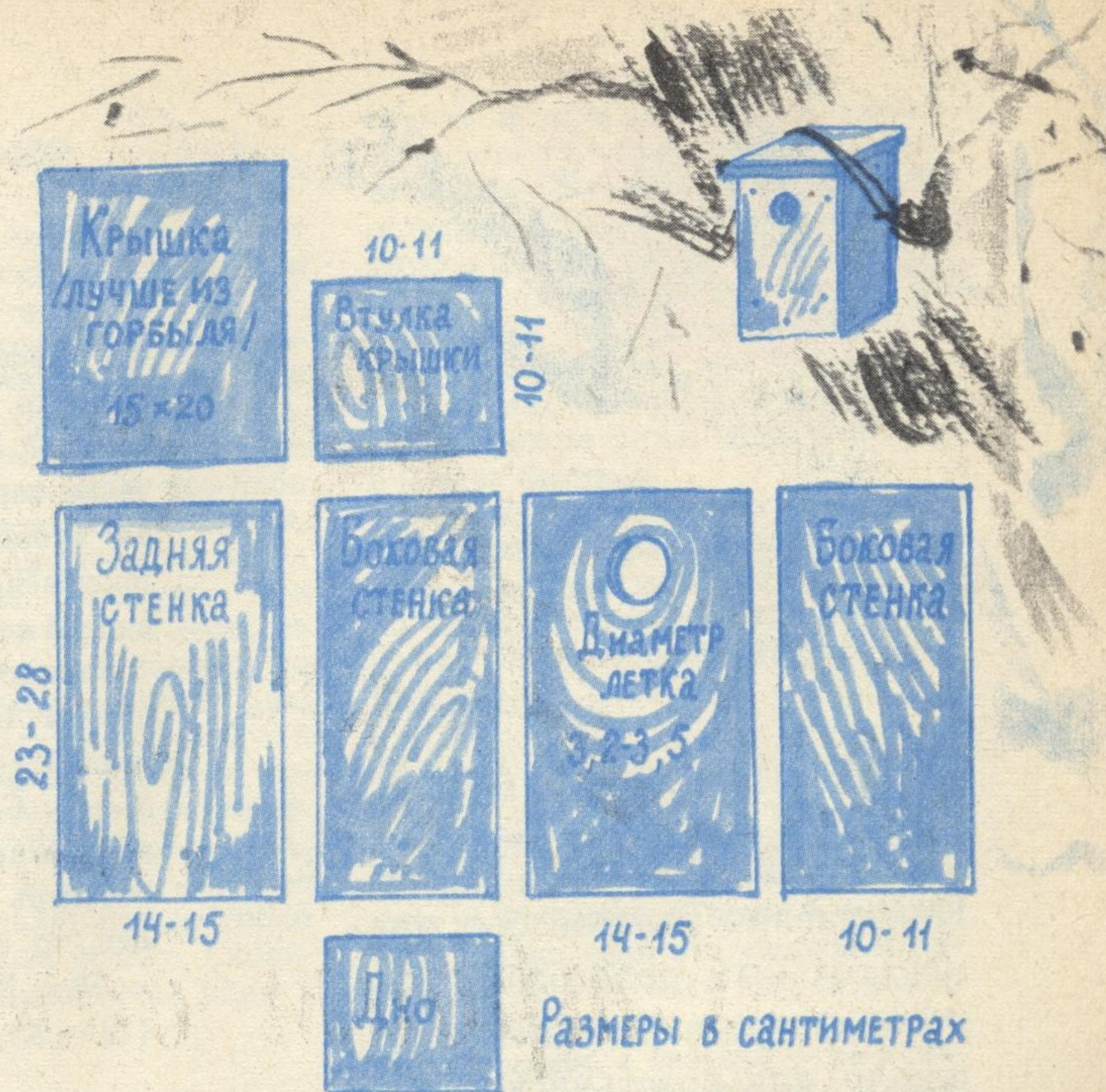
РАЗМЕРЫ ПТИЦЫХ ДОМИКОВ
