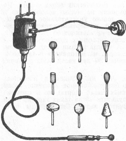
Электродвигатель с гибким валом и набором фрез и камней для шлифовки каналов.
