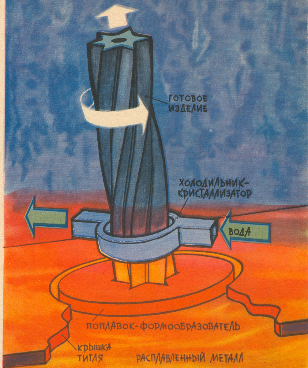
ПОЛУЧЕНИЕ ВИТОЙ РЕБРИСТОЙ ТРУБЫ ИЗ РАСПЛАВА
