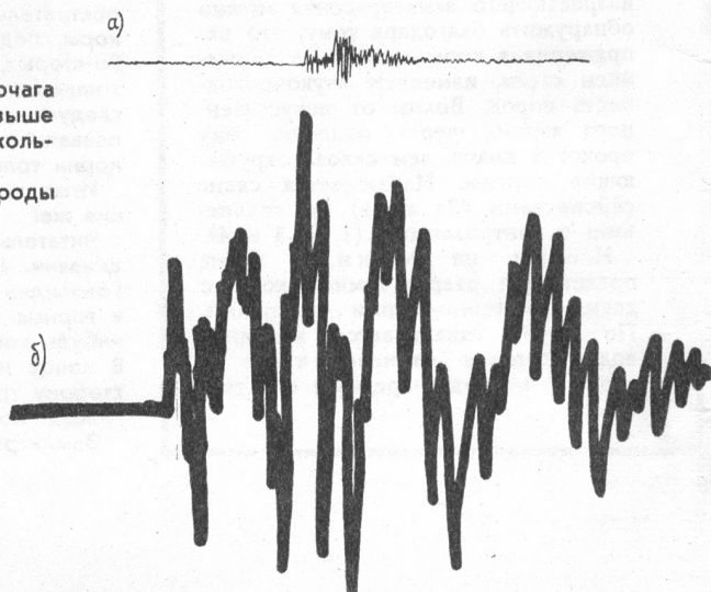
График повторяемости позволяет предвидеть частоту грядущих землетрясений. а) Запись очень слабого землетрясения прибором с увеличением в 100 тыс. раз. б) Запись сильного землетрясения прибором с уменьшением в 2 раза.
