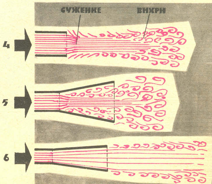
СХЕМА ИСТЕЧЕНИЯ ОТРАБОТАННЫХ ГАЗОВ ИЗ ВЫПУСКНЫХ ТРУБ
