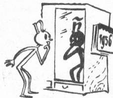
В 1956 году была открыта нейтральная античастица.
