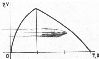
Изменение давления газа и скорости снаряда в зависимости от времени и пути его.
