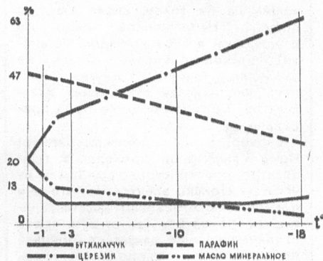
Зависимость содержания основных компонентов лыжной мази при отрицательной температуре воздуха.
