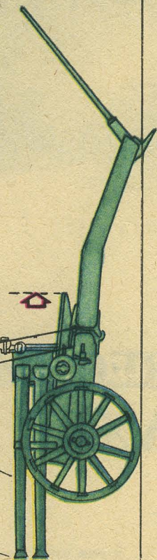
215. Шведское 81/37-мм пехотное орудие системы «Бофорс». Масса снарядов 4,4/0,7 кг, начальная скорость снарядов — 320/800 м/с, угол возвышения стволов — 8—80°, дальность стрельбы — 6000/7100 м.
