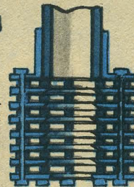
Д. Устройство дульного тормоза системы «Шнейдер».
