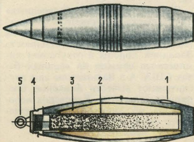
Американский 203,2-мм химический снаряд М426: 1 — предохранитель ведущего пояса, 2 — разрывной заряд, 3 — отравляющее вещество, 4 — переходная втулка, 5 — холостая пробка с ушком.
