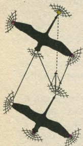
Полетный строй гусей. Модельные эксперименты позволяют представить соотношение электрических полей и кулоновых сил.
