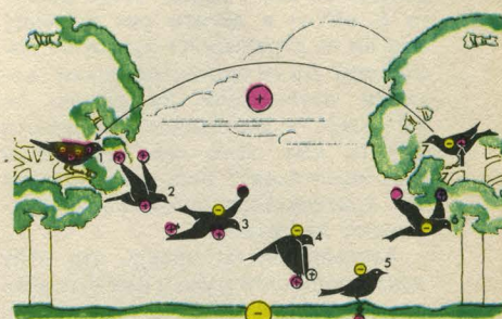
Так происходит электрическая зарядка и поляризация птицы. 1, 5, 7 — при контакте с земной поверхностью свободные электрические заряды нейтрализуются. 2, 3, 4, 6 — в процессе полета вырабатывается высокий электростатический заряд.
