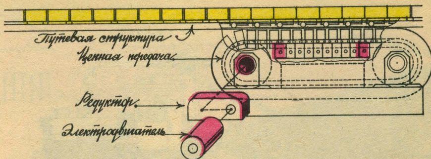
Привод поточно-конвейерной системы.
