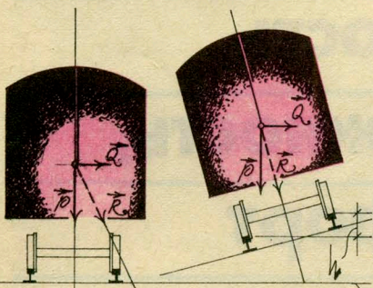
Схема расчета величины превышения внешнего рельса на поворотах.
