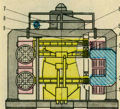
Новый роторный сепаратор. Цифрами обозначены: 1 — блок катушек, 2 — магнитопровод, 3 — электромагнитная система, 4 — блок роторов, 5 — дополнительный верхний полюс, 6 — рама, 7 — привод, 8 — питатели, 9 — ферромагнитные пластины.
