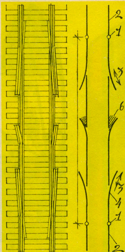
Стык «бархатного» пути: 1 — начало компенсирующей линейное расширение вставки, 2 — рельсовая плеть, 3 — направления перемещений вставки, 4 — перемещающиеся усовики рельсовых плит, 5 — уравнильная вставка, 6 — изолирующее соединение.
