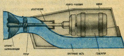
Переносная микроГЭС.
