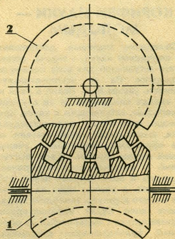
Бесконтактная червячная передача: 1 — червяк, 2 — зубчатое колесо.
