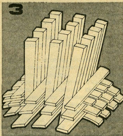
Трехмерно армированный каркас в цилиндрической системе координат.
