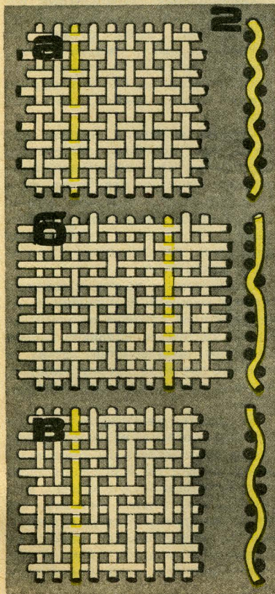
Переплетение нитей в трикотажных сетках.
