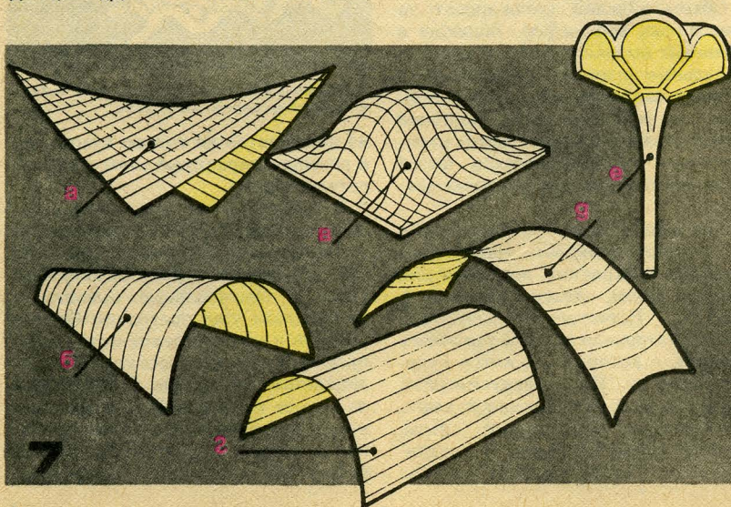
Различные виды оболочек: А — гиперболический параболоид, Б — купол, В — двоякоизогнутая конструкция, Г — коноид, Д — цилиндр, Е — лепестковая оболочка.
