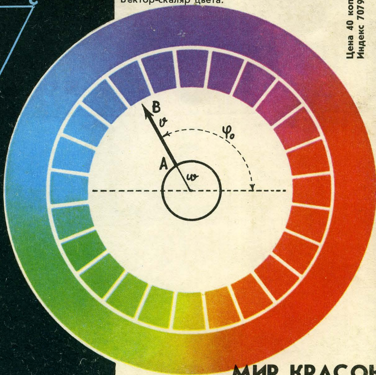
Вектор-скаляр цвета.
