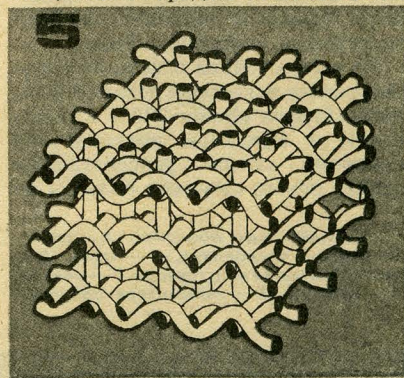
Образец плетения многослойных тканей в композиционном материале.
