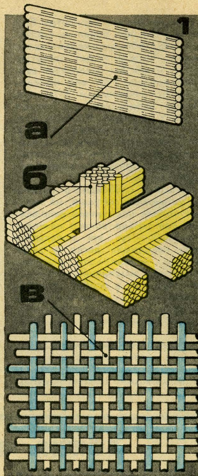
Схемы армирования композиционных материалов при прямоугольной укладке волокон: А — одно-, В — двух- и С — трехмерные структуры.
