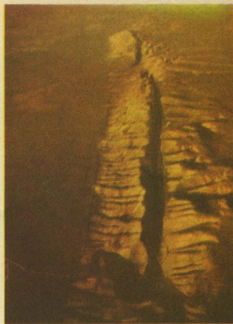
Сейсмоактивный район — граница Тихоокеанской и Американской литосферных плит в долине Сант-Андреас в Калифорнии.
