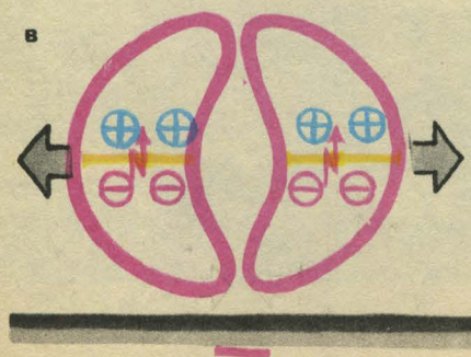
Рис. 3. Движение зарядов в расширенном участке разряда между облаком и землей (а), спутный разряд ионов и электронов (б) и возникшая ШМ (в).
