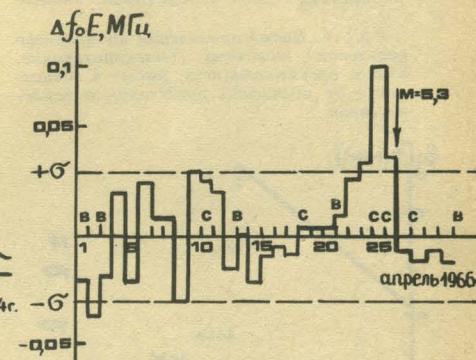
Рис. 5. Среднесуточное отклонение критической частоты ионосферного слоя E перед Ташкентским землетрясением. Буквами обозначены магнитовозмущенные (В) и магнитоспокойные (С) дни; ~ — среднеквадратическое отклонение критической частоты.
