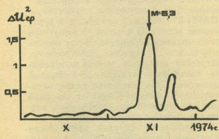
Рис. 3. Усредненные реализации возмущений электротеллурического поля в районе Киятлинского землетрясения (Кавказ).
