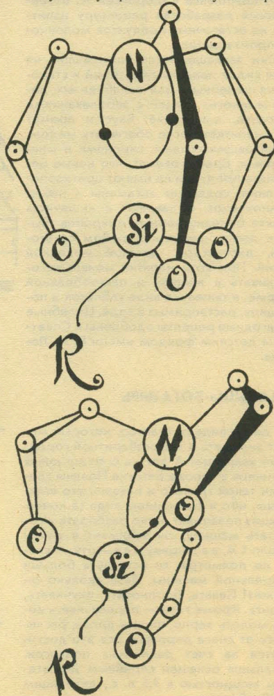
Рис. 1. Новый тип кремнийорганических гетероциклов — силатраны. Структура молекулы показана в двух ракурсах. Две точки внутри атомарной «клетки» — неподделенная пара электронов атома азота. R — углеводородная или другая группа.
