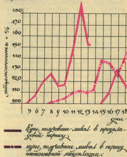
Рис. 3. Влияние мивала и мигуена на яйценоскость кур. Сплошная линия — скармливание мивала перед яйцекладкой; штрихпунктир — в период интенсивной яйцекладки.
