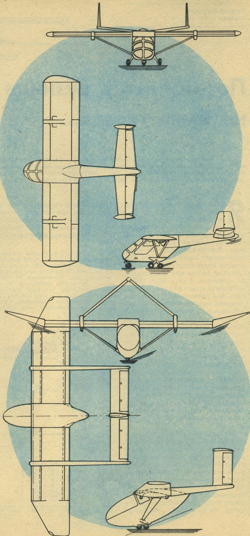
Рис. 4. Самолет для СЛА. Берите на заметку!
