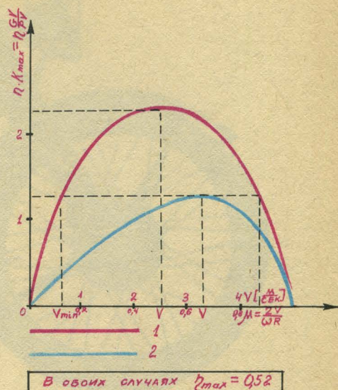
Рис. 5. Сравнение кривых эффективности ( K_{max} ) обычного винтового (2) самолета и машины Болдырева (1). Обозначения: M — отношение скорости потока от предкрылка или винта к скорости набегающего потока; \eta — КПД силовой установки; G — полный вес аппарата или переносимой им полезной нагрузки; V — скорость перемещения груза; P — сила тяги, развиваемая силовой установкой; n — частота колебаний.
