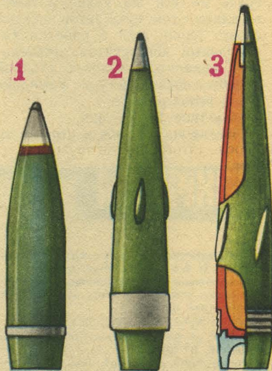
1 — современный снаряд традиционного типа, 2 и 3 — современные снаряды с готовыми выступами.
