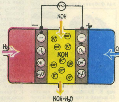
Рис. 2. Основные электрохимические процессы в топливном элементе.
