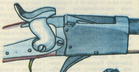
93. Австрийская пехотная винтовка системы Венцеля образца 1867 года под патрон бокового боя. Длина со штыком — 1810 мм, длина без штыка — 1330 мм, длина ствола — 880 мм, калибр — 14,5 мм.
