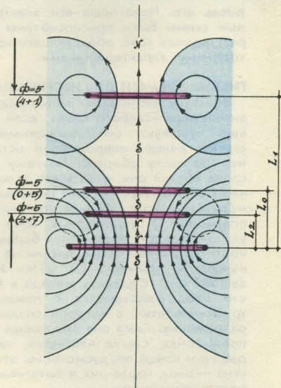
Рис. 2. Три положения идеальнопроводящих колец. \Phi — число силовых линий, в скобках — сумма силовых линий, принадлежащих меньшему и большему кольцам.
