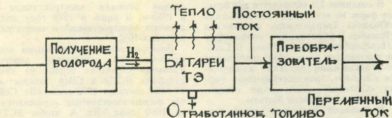
Рис. 3. Принципиальная схема электростанции на топливных элементах.
