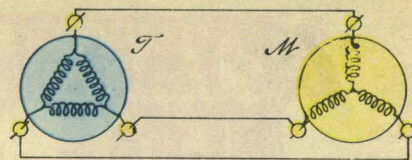
Рис. 7. Система, созданная Доливо-Добровольским.
