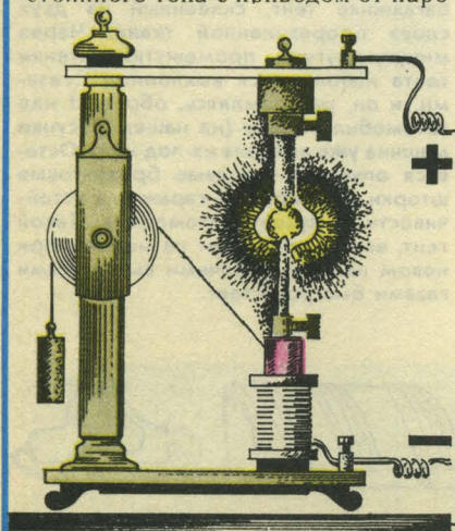
Рис. 1. Регулятор Аршро.
