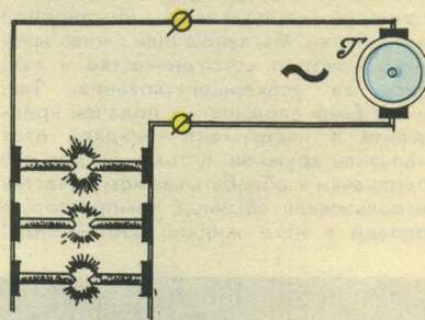
Рис. 3 Первоначальная схема подключения «свечей Яблочкова».
