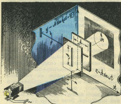
Рис. 6. Модель для демонстрации сложения двух гармонических колебаний.
