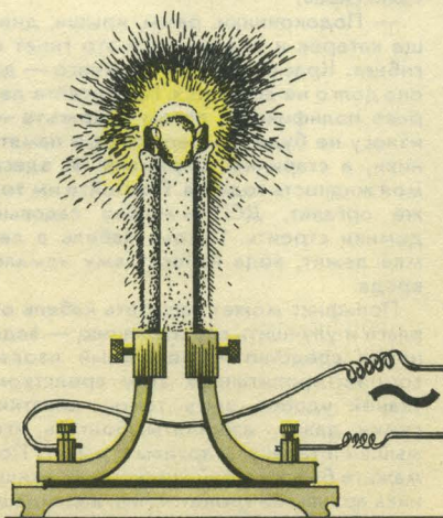
Рис. 2. «Свеча Яблочкова».
