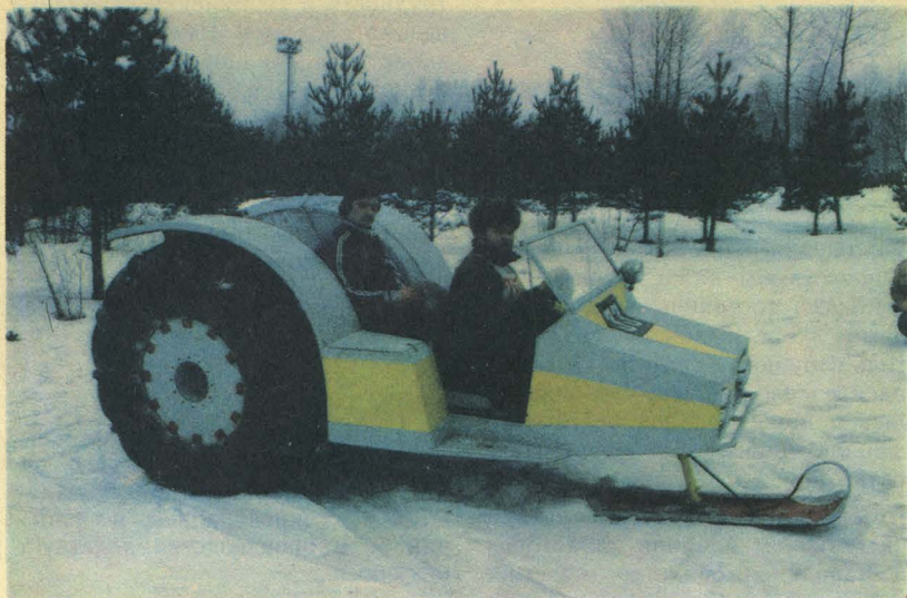
Один из победителей III Всесоюзного смотра-конкурса самодельных вездеходов на пневматиках низкого давления — вездеход В. Андрианова и А. Никитина (г. Ярославль), удостоенный почетного диплома «Техники — молодежи». Фото С. КОСЬЯНОВА.
