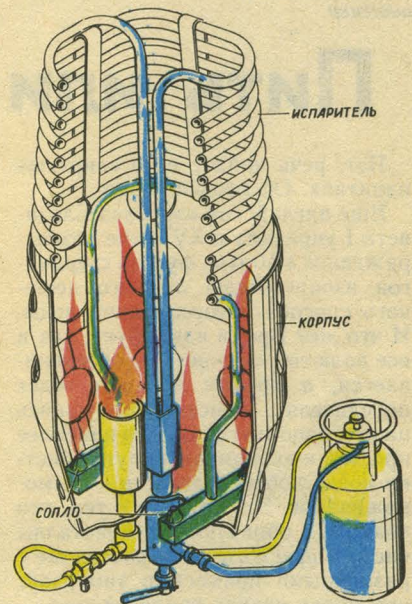
Устройство наиболее распространенного генератора тепла.
