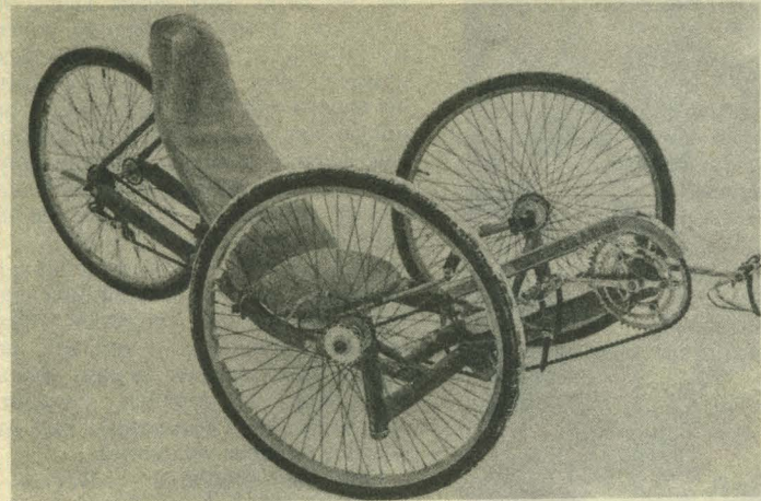
Велосмобель «Крузиз» — образец классической конструкции. Вес — 18 кг, максимальная скорость — 30 км/ч.
