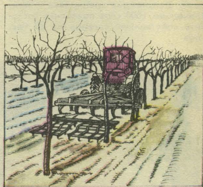
Для разравнивания почвы между саженцами можно применить тракторный плуг, у которого от отвала переднего корпуса приделан удлинитель из листовой стали, которому придана форма полуцилиндра. Его размеры — длина 1050 мм, ширина — 500 мм, толщина — 3 мм.
