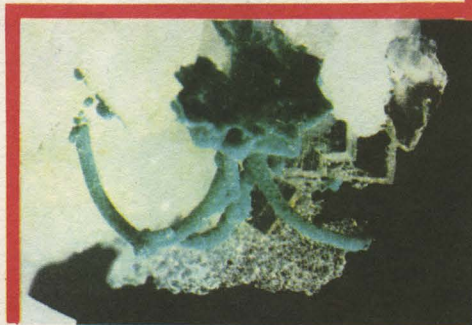
вверх: малахит, розовый гематит, оливинит, барит.
