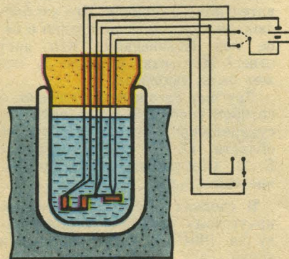
Схема установки 1959 года, предложенная комиссией президиума АН СССР.
