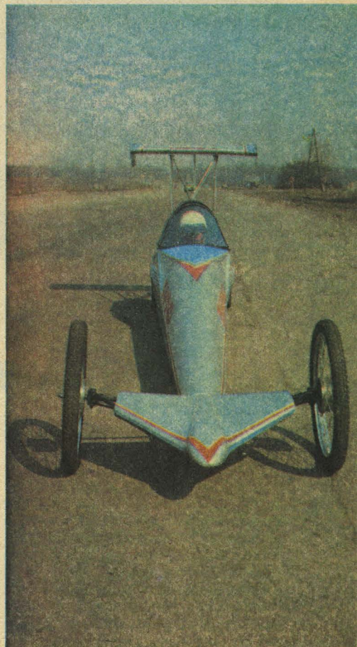
Еще один представитель династии харьковских рекордсменов — электрокар ХАДИ-13Э.
