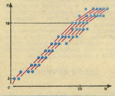
График зависимости числа протонов от числа нейтронов для ядер четных элементов.
