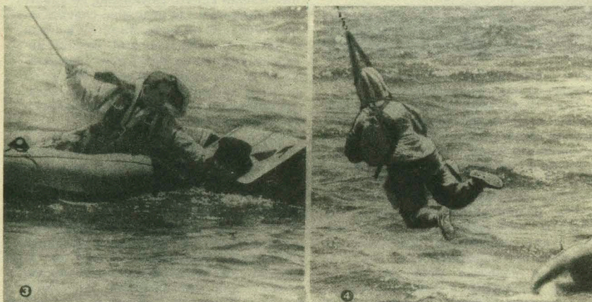
Система «Небесный крюк» в действии: 1 — летчик, находясь в надувной спасательной лодке, надев подвесное устройство, заполняет гелием мини-аэростат, 2 — аэростат готов к запуску, 3 — летчик освобождается от шлюпки, 4 — начинает «вознесение на небо», 5 — еще несколько секунд, и экипаж самолета-спасателя втянет его в кабину.
