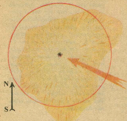
Рис. 1. Форма зоны лесоповала в районе Тунгусской катастрофы. Показан круг, площадь которого равна площади зоны; его центр — точка пересечения линий повала отдельных деревьев. Стрелка — проекция скорости пролета космического тела на земную поверхность (по В.А. Золотову).
