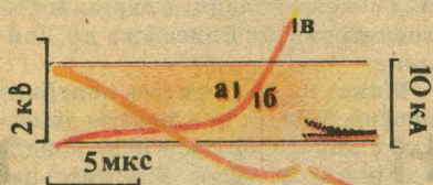
Рис. 2. Осциллограммы тока и напряжения, полученные в процессе электрического взрыва медного проводника; а и б — начало и конец его плавления, в — начальная точка взрыва.
