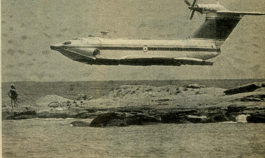
Со скоростью 330 км/ч «Орленок» несется в двух метрах над водой.
