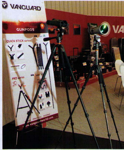
Обыденное применение углепластиков, конечно, не ограничивается рукоятками ножей. Штатив для фотоаппаратов и других оптических приборов, изготовленный из углепластика (справа) при одинаковой величине, прочности и жёсткости весит в 1,5 раза меньше, чем изготовленный из сплавов лёгких металлов, например дюралюминия (слева). Дополнительное преимущество это неизменный в процессе эксплуатации внешний вид, тогда как каждая царапина и каждая потёртость на чёрном анодированном покрытии дюралюминиевого штатива будут буквально бросаться в глаза своим серебристым блеском.
