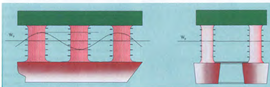
Схема полупогруженной морской платформы повышенной волнотойкости с двумя погруженными понтонами
