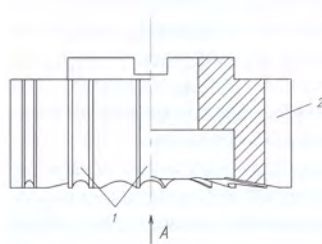
Рис. 9. Реверсивная торцовая фреза. 1 – двухсторонний режущий зуб; 2 – стружкоотводная канавка
